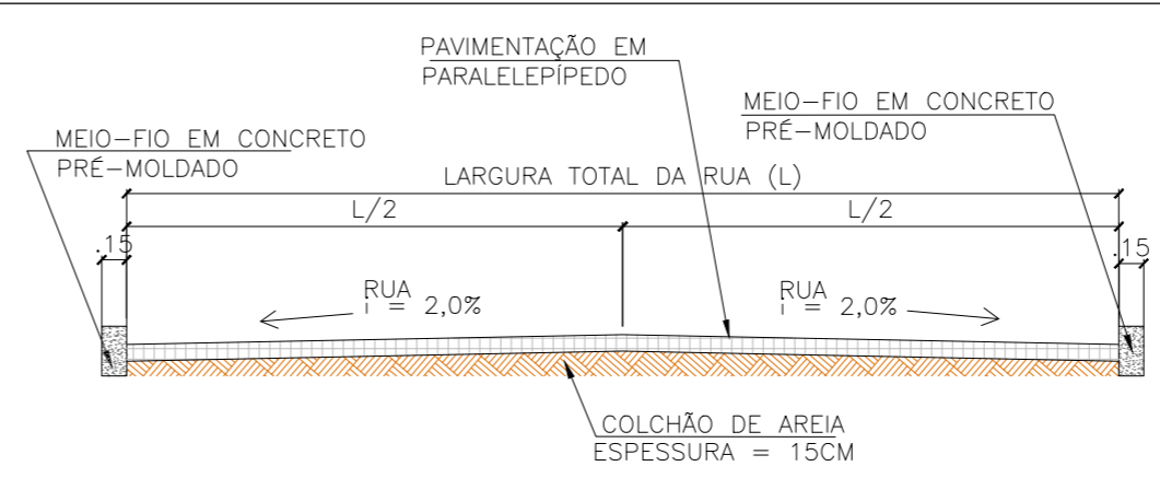
CORTE TRANSVERSAL - TRECHO 12 Pavimentações, Jucurutu/RN Sem escala
