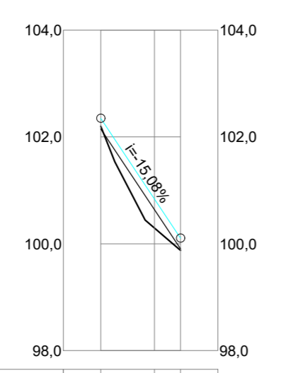
TRECHO 12-SERRA DO JOAO DO VALE - E00 ATE E00+14,88m PERFIL LONGITUDINAL - ESC.: V=1:100 H=1:1000
